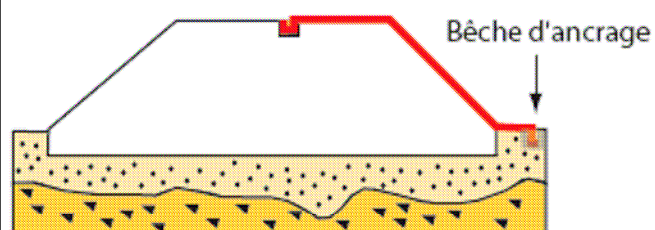
2 Complexe d'étanchéité amont
