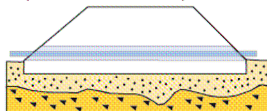
8 Canalisation de vidange et enrobage de la conduite par du béton coulé pleine fouille afin d'éviter l'apparition de renards
