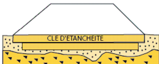
3 Clé d'étanchéité
