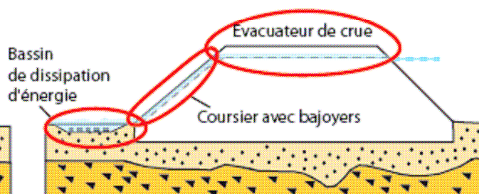
10 Surverse, bajoyers et bassin de dissipation d'énergie
