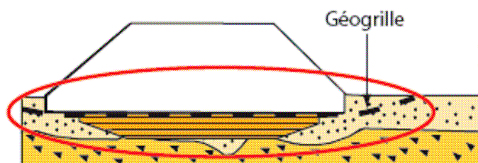
5 Purge et substitution du sol réduite + géogridde pour assurer la portance du sol
