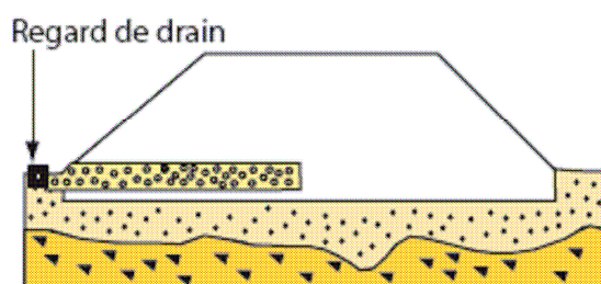
6 Drain horizontal pour évacuer l'eau du corps de remblai
