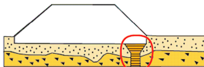
9 Coupure d'étanchéité en cas de fondation perméable
