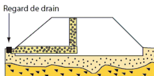
7 Drain vertical + horizontal pour évacuer l'eau du corps de remblai
